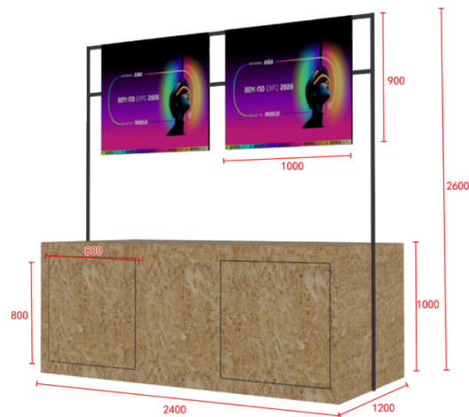
圖表3：初創展位設計圖
