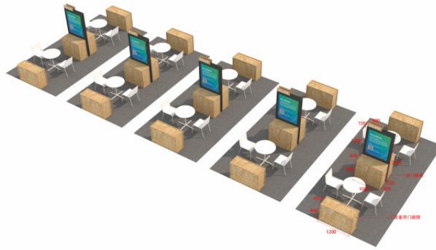
圖表2：標準展位設計圖
